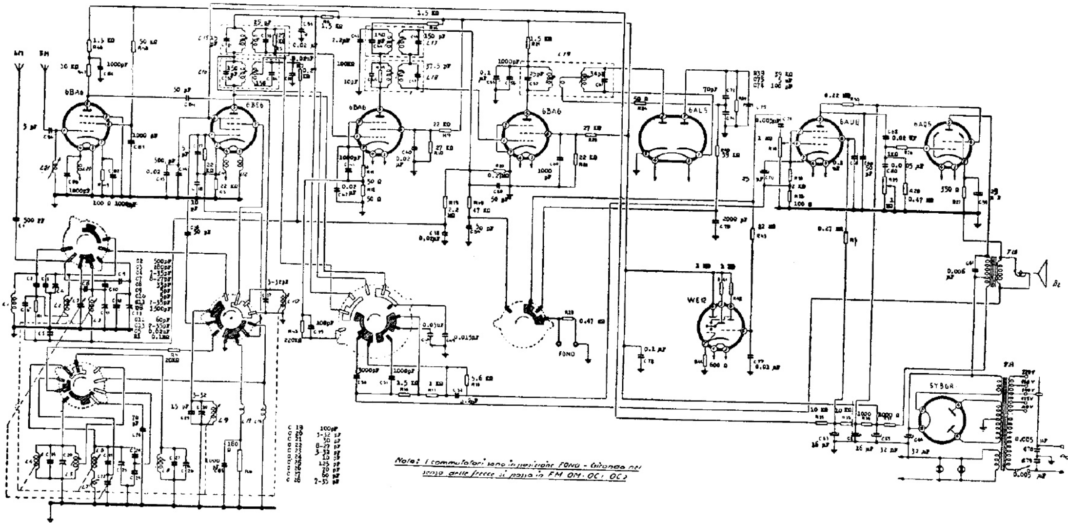
TELEFUNKEN (COMPAGNIA RADIORICEVITORI) - Mod. T 84 FM - A modulazione d'ampiezza e di frequenza. Media frequenza per AM 468 kc; media frequenza per FM 10,5 Mc. La 6BE6 provvede alla conversione per l'AM e per l'FM. La seconda 6BA6 amplifica la MF per l'AM e per l'FM; la terza 6BA6 provvede alla rivelazione AM e alla seconda MF/FM.
